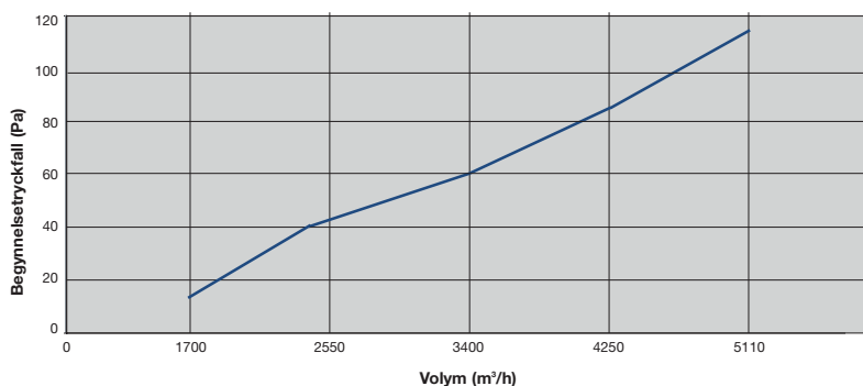
Tryckfall Pa vid olika flöden*
