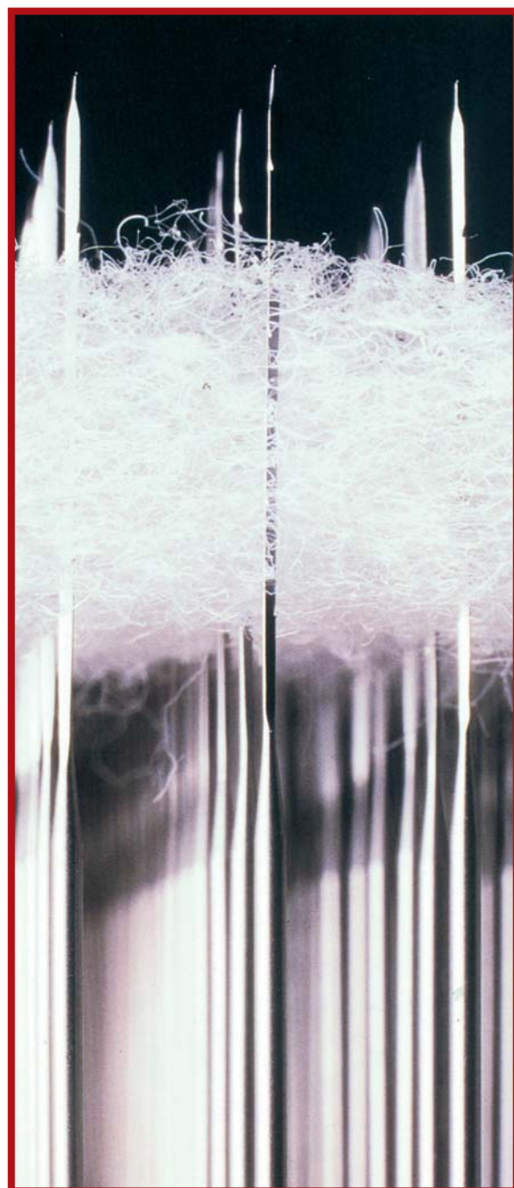
Fig 7. Hullingsförsedda nålar binder fast fibrerna i varandra och i basväven.
