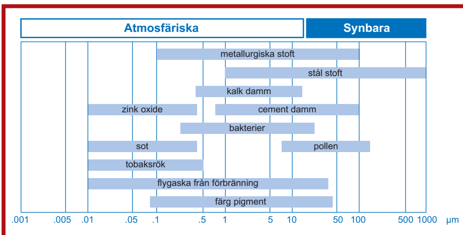
Fig 3. Klassificering av stoftpartiklar.
